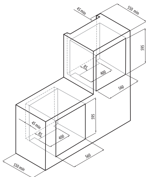
Рис. 5. Схема ниши для встраивания духового шкафа
