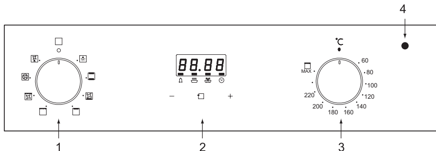
Рис. 1. Панель управления
