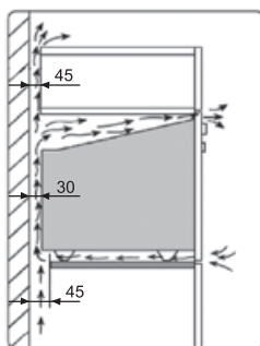
Рис. 6. Схема по встраиванию духового шкафа
